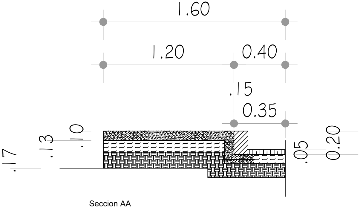
Seccion AA
