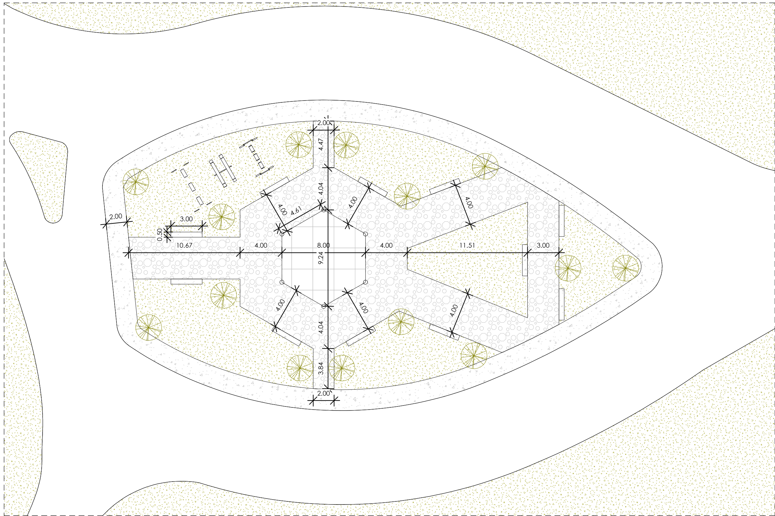
1 PLANTA ARQ. DIMENSIONADA AQ-02 1 : 225
