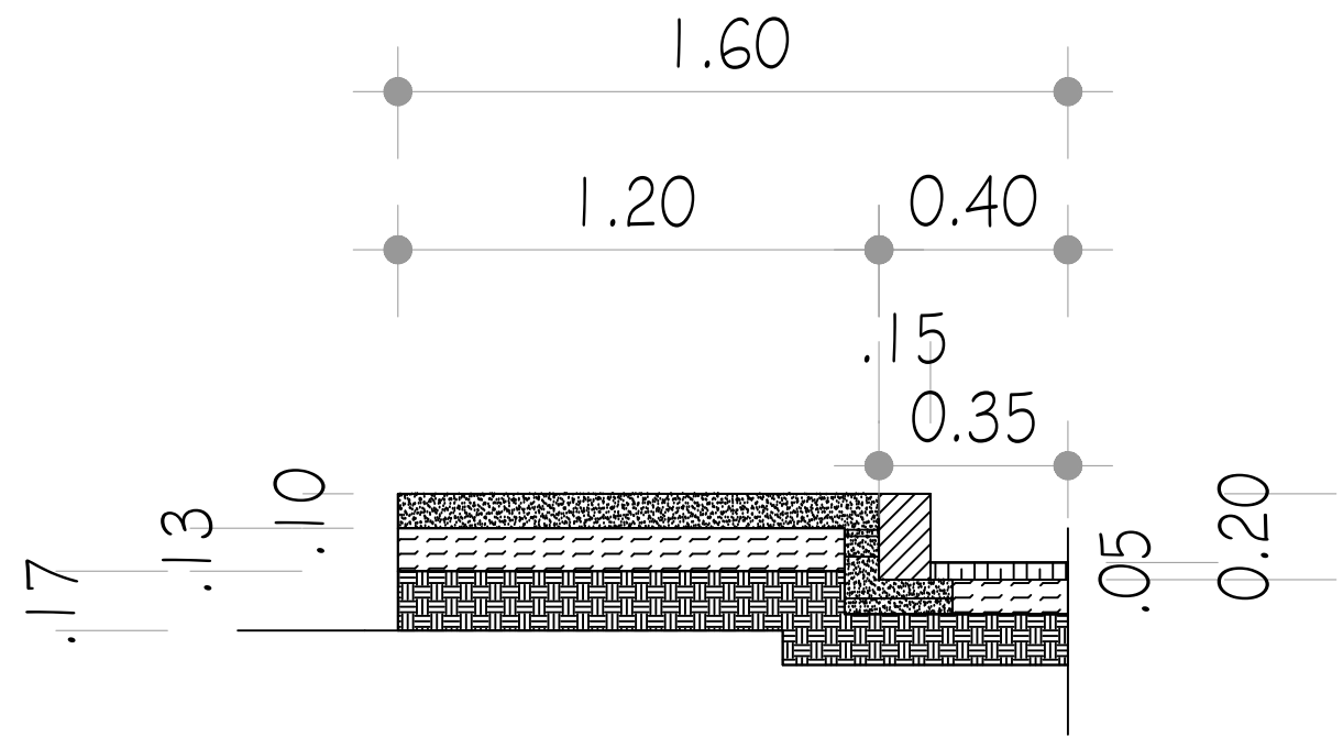
Seccion AA
